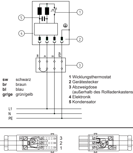
Fig. 5 Schaltbild RolTop-868 230 V / 50 Hz und Kabelbelegung bei Verwendung mit Hirschmann-Steckverbindung STAS-3 (mit Brücke)
