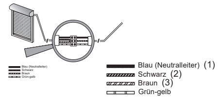
Fig. 7 Anschluss Funk (Senderbetrieb)
